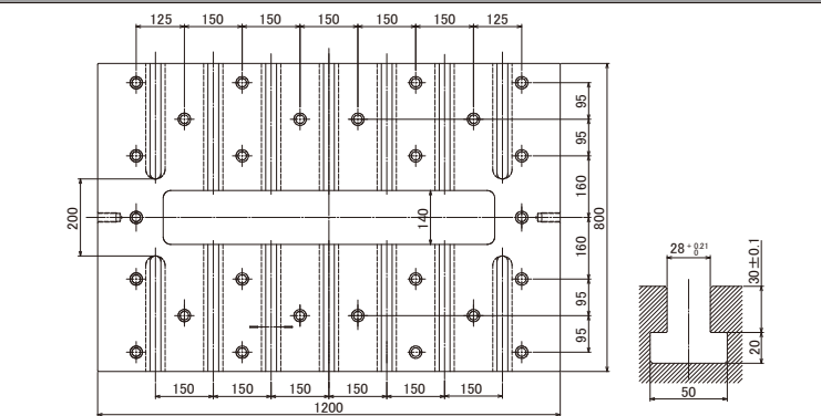
工作台 / Bolster
