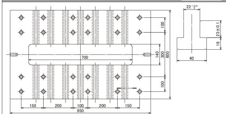
工作台 / Bolster
