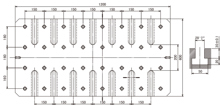
工作台 / Bolster
