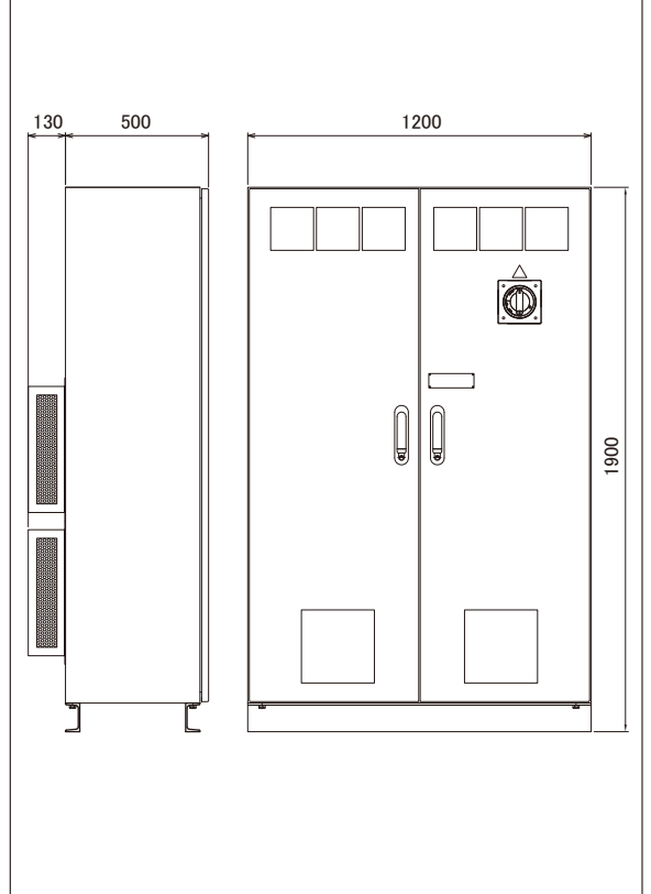
控制箱 / Control Box
